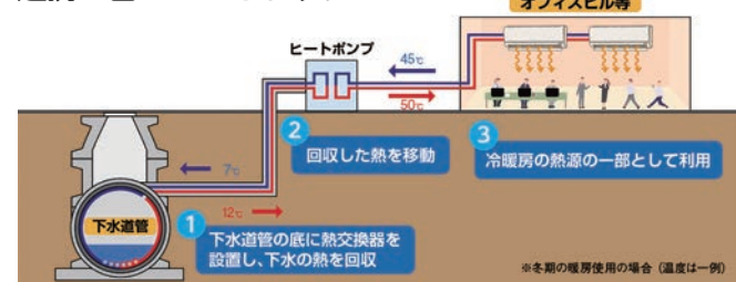
下水道管からの熱利用（イメージ）
