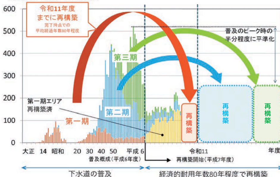
下水道管の年度別整備延長(km)
