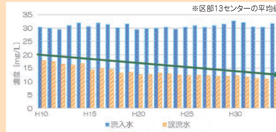
区部水再生センターの放流水質（全窒素）※の経年変化
