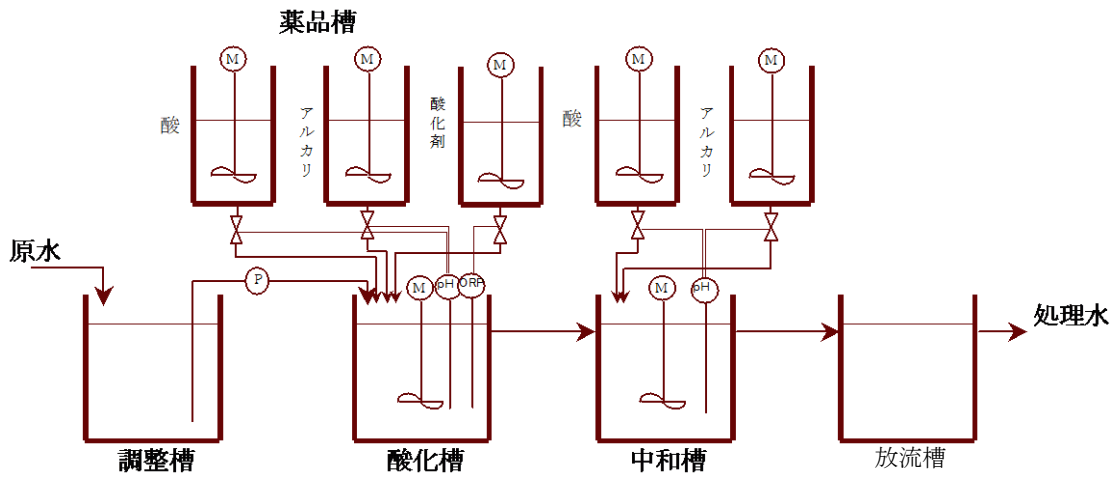
図 2 - 1 6 薬品酸化法
