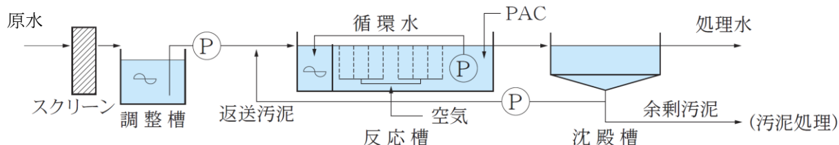
図2-22 嫌気好気活性汚泥法
