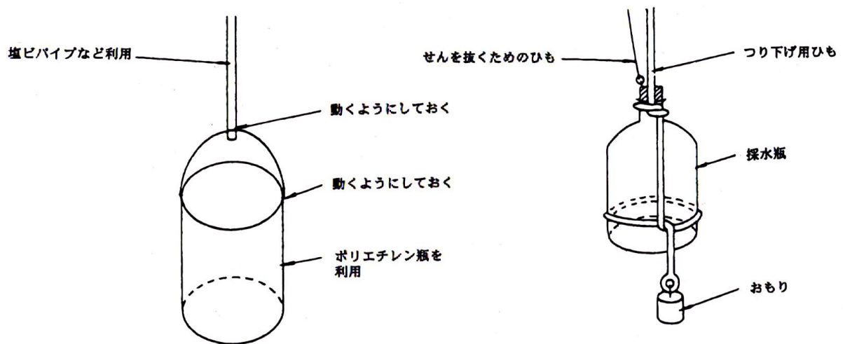
図5-2 簡易採水器
