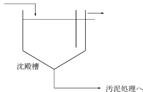
図2-3 自然沈殿法
