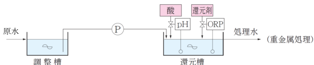
図2-9 還元法
