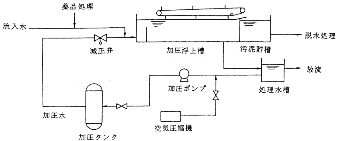
図6-2 加压浮上法
