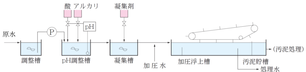
図2-4 加圧浮上法
