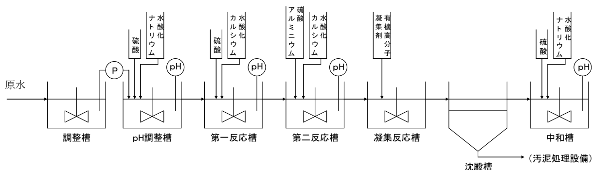
図 2 - 1 5 ふっ素処理
