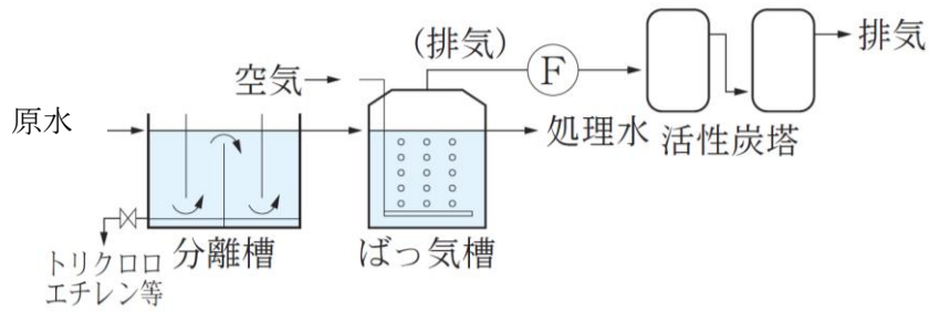
図 2-20 ばっ気法
