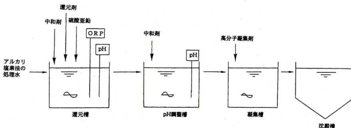
図2-8 亜鉛白法
