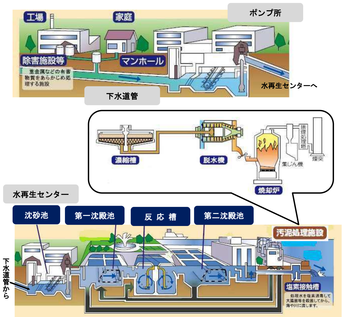
図2-4 下水処理のしくみ
