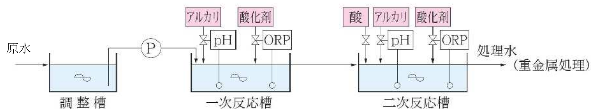
図2-7 アルカリ塩素法
