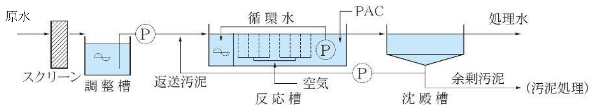
図 2-22 嫌気好気活性汚泥法
