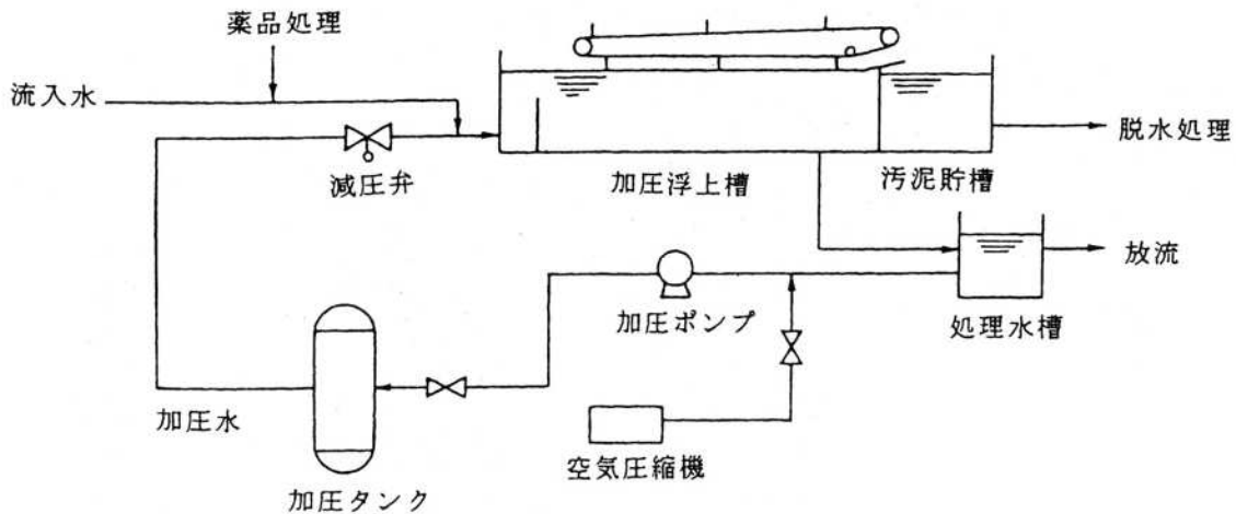
図 6 - 2 加压浮上法
