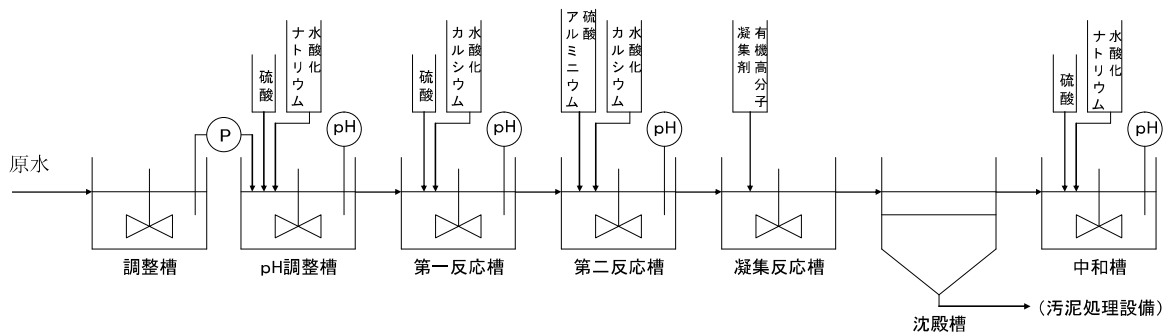
図 2-15 ふっ素処理
