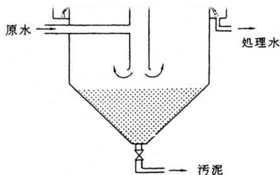
図6-1 沈殿槽
