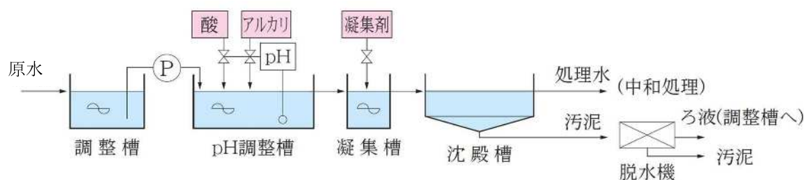
図 2-10 凝集沈殿法
