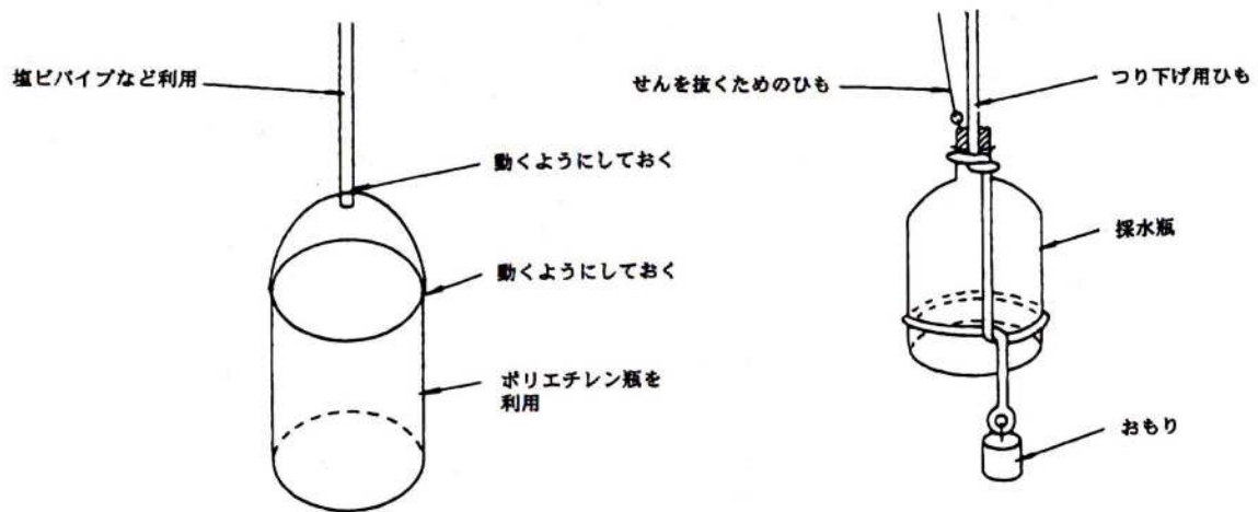
図5-2 簡易採水器
