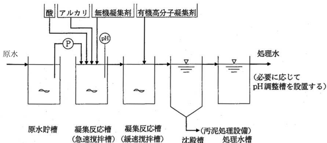
図2-4 凝集沈殿法
