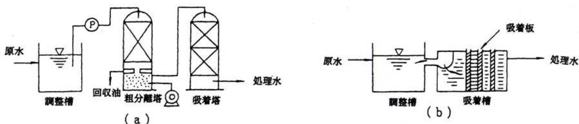
図2-5 吸着法
