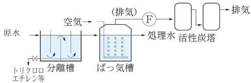
図 2-20 ばっ気法
