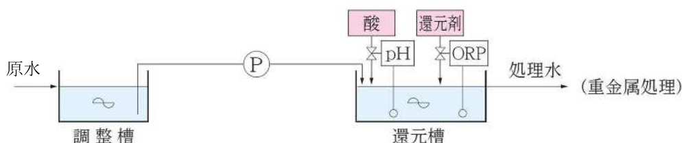
図2－9 還元法
