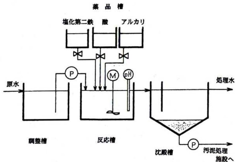
図 2 - 1 7 凝集沈殿法
