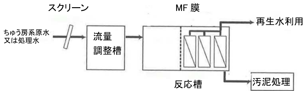
図 6 - 5 膜分離活性汚泥法
