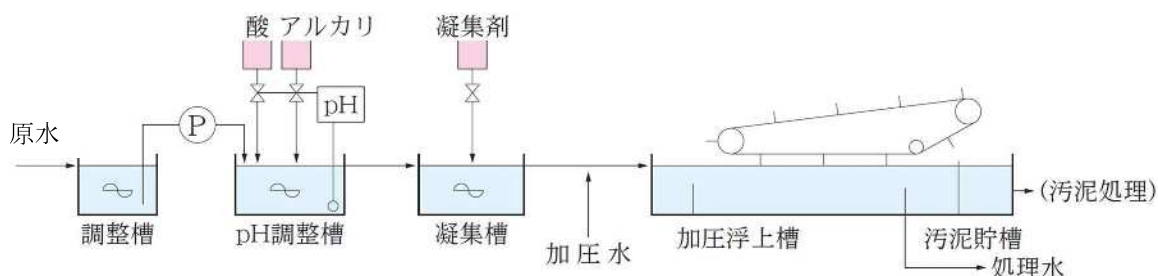
図2-4 加圧浮上法
