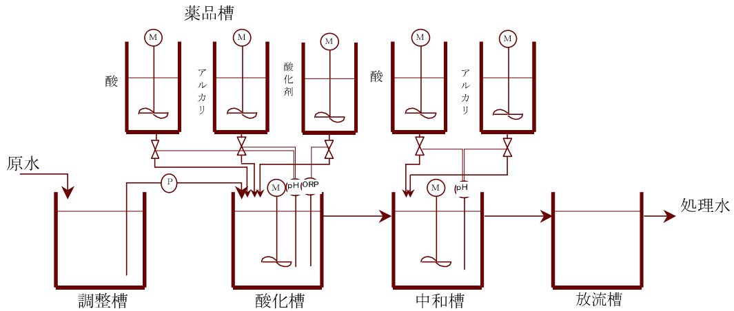
図 2 - 1 6 薬品酸化法
