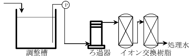
図 2-13 イオン交換法
