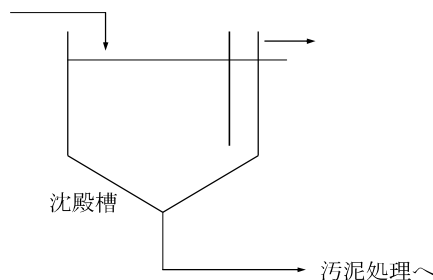
図2-3 自然沈殿法
