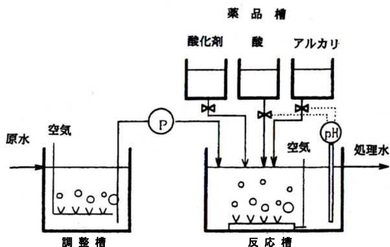
図 2-18 空気酸化法
