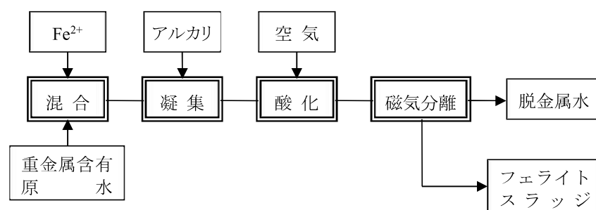
図2-11 フェライト法
