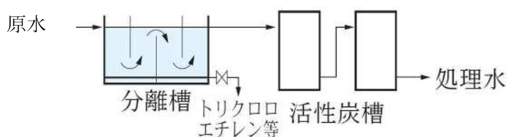
図 2-19 活性炭吸着法
