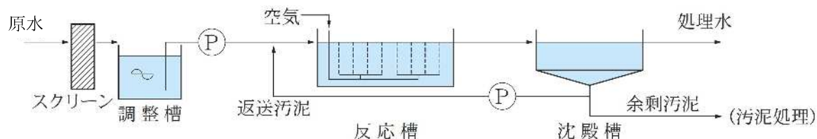
図2-6 活性汚泥法
