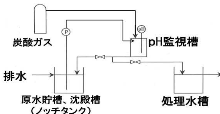
図2-2 炭酸ガス中和法
