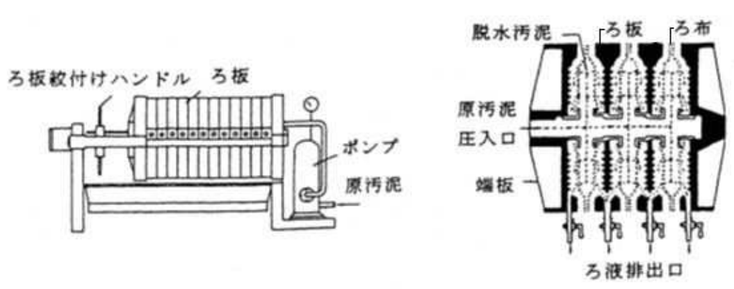
図6-3 フィルタープレス
