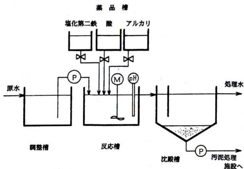
図 2 - 1 7 凝集沈殿法
