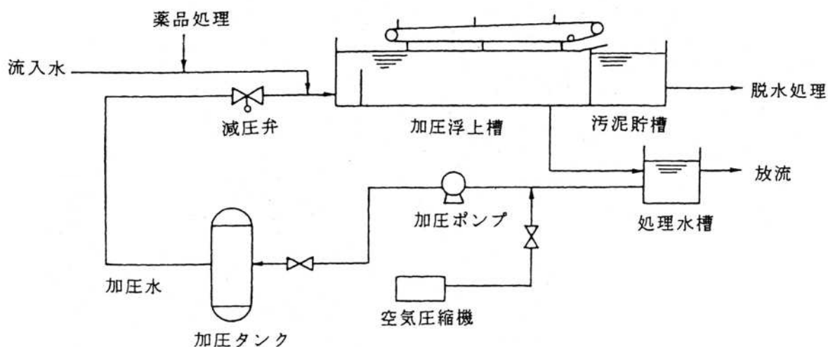
図 6 - 2 加压浮上法
