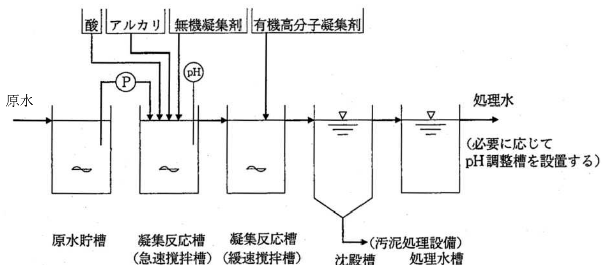
図2-4 凝集沈殿法
