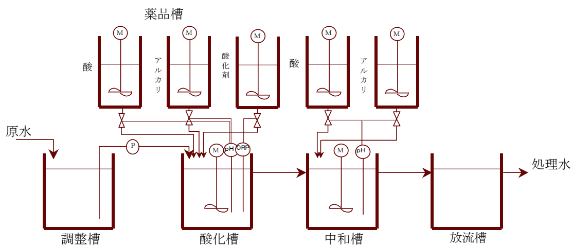
図 2 - 1 6 薬品酸化法
