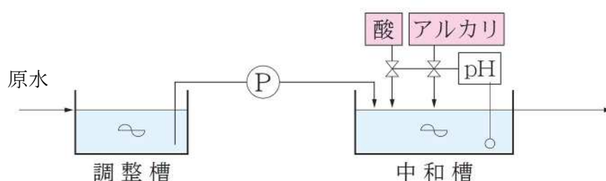
図2-1 連続式中和法
