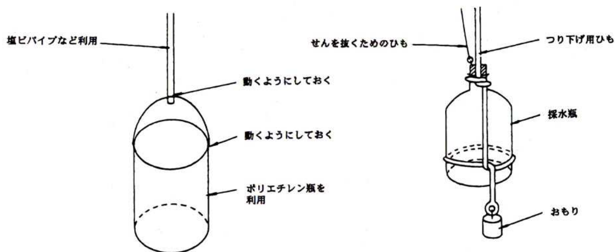
図 5 - 2 簡易採水器
