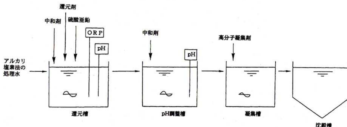
図2-8 亜鉛白法
