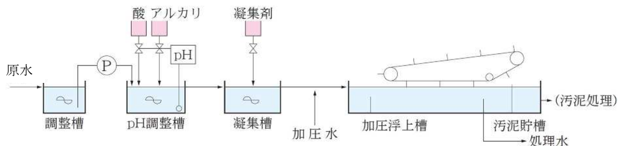
図2-4 加圧浮上法
