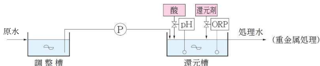
図2－9 還元法
