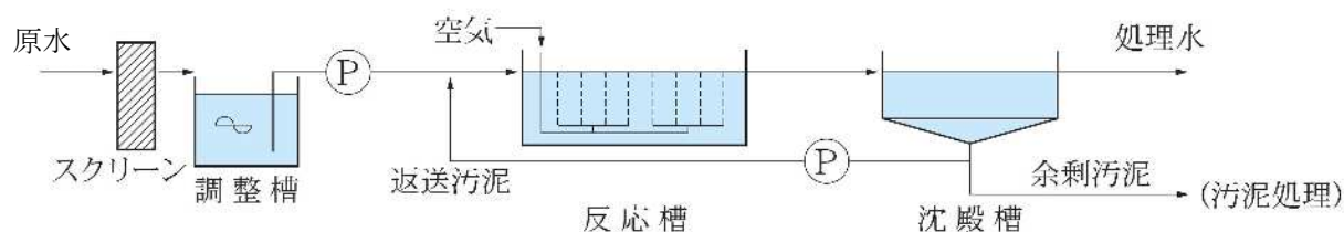
図2-6 活性汚泥法
