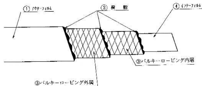
図 2-2-1 取付管ライナー構造図
