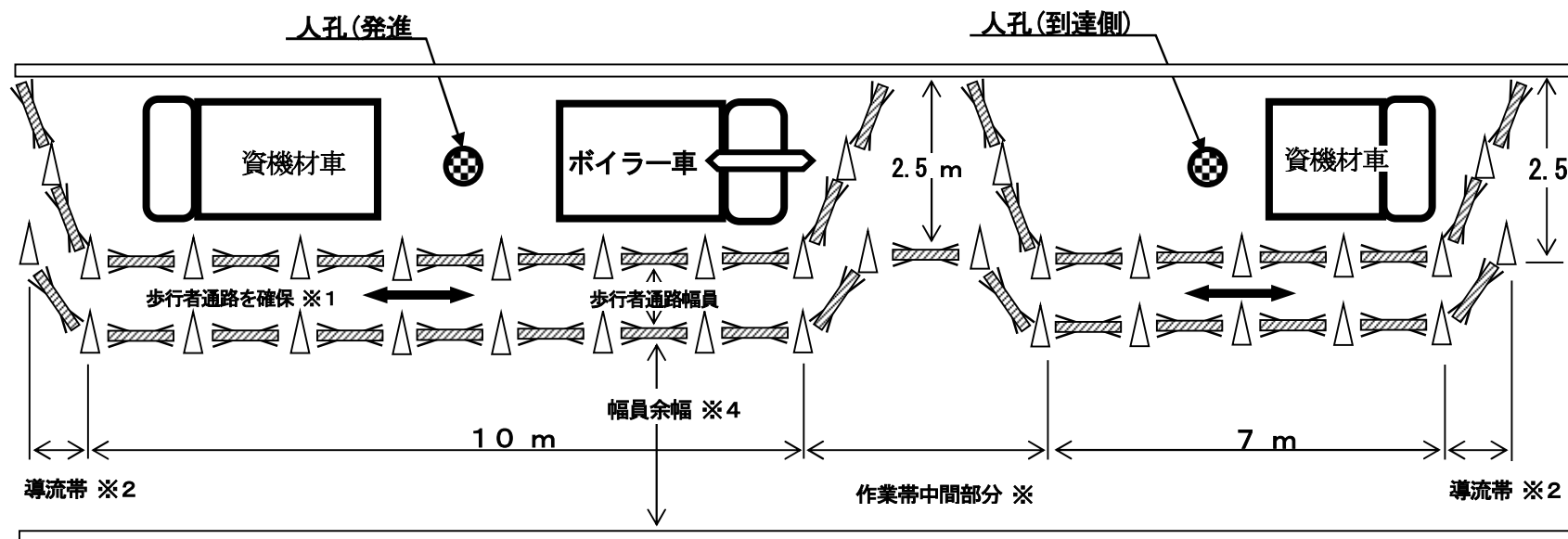
図1-5-3 蒸気硬化
