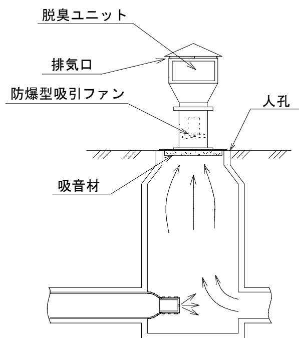
図 3－1 脱臭・防音装置
