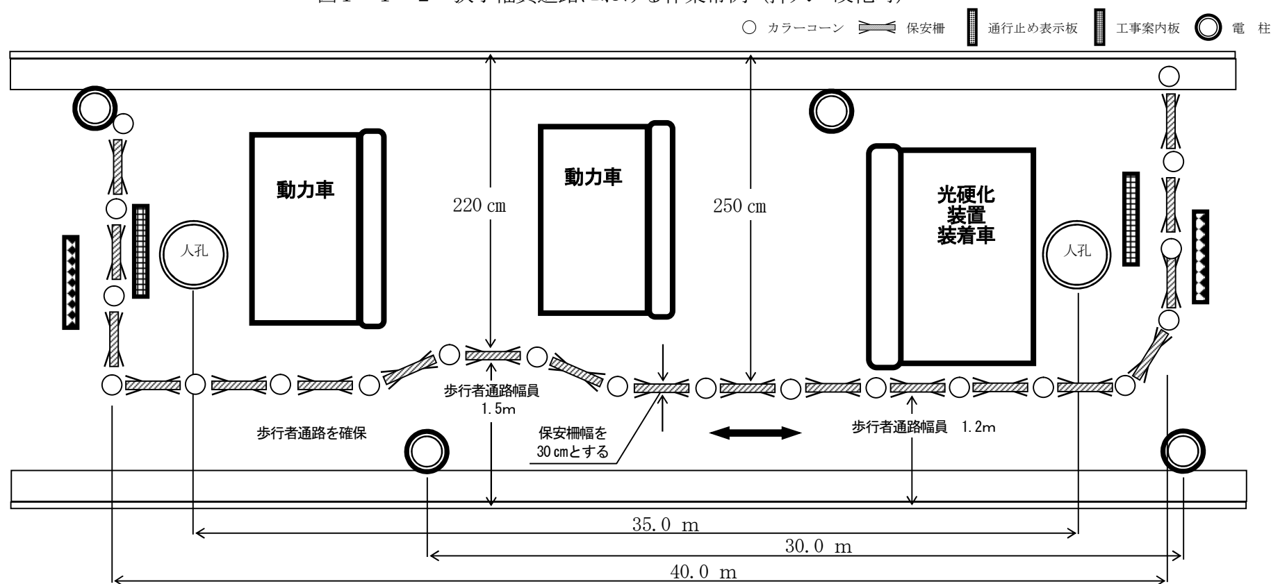
図1-1-2 狭小幅員道路における作業帯例（挿入・硬化時）
