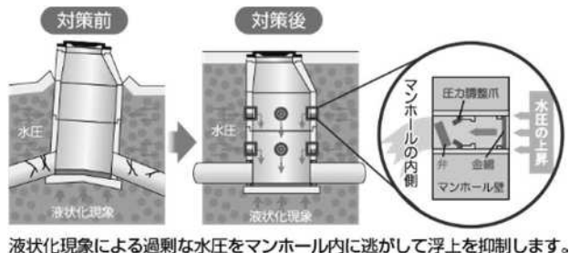
図表2-24 マンホールの浮上抑制対策
