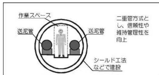
図表2-28 送泥管の再構築のイメージ図
