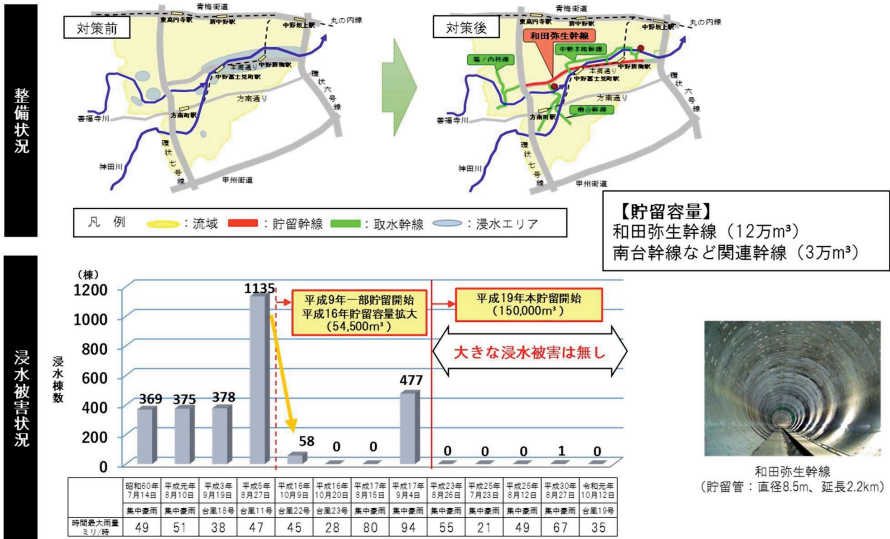
図表 2-7 和田弥生幹線の整備効果
