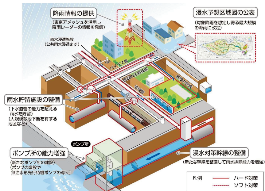
図表 2-3 浸水対策のイメージ
