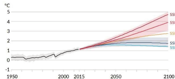
図表 2-16 今後予測される世界平均地上気温の変化（IPCC 第6次評価報告書）
