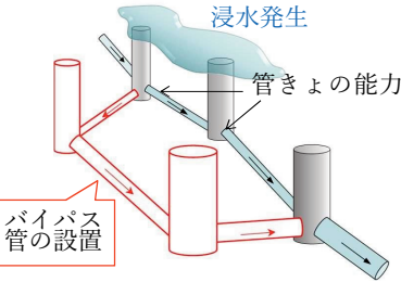
小規模なバイパス管の設置
