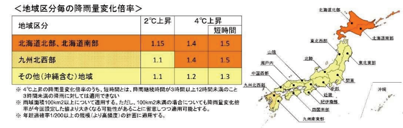
図表 2-18 地域区分毎の降雨変化倍率
