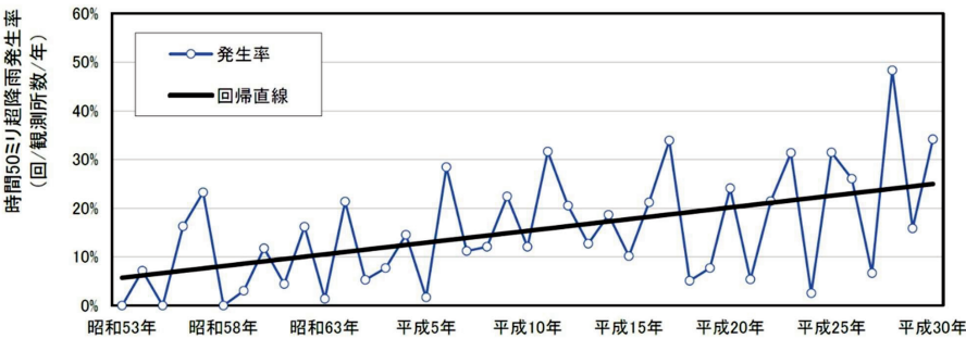
図表 2-10 都内における 1 時間 50 ミリを超える豪雨発生率の推移 データ出典：東京都建設局「過去の水害記録」
