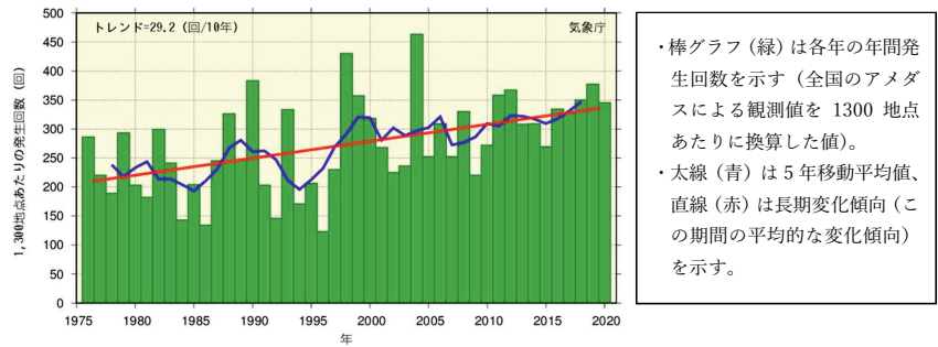
図表 2-9 全国（アメダス）1 時間降水量 50 ミリ以上の年間発生回数 出典：気象庁ホームページ「大雨や猛暑日など（極端現象）のこれまでの変化」
