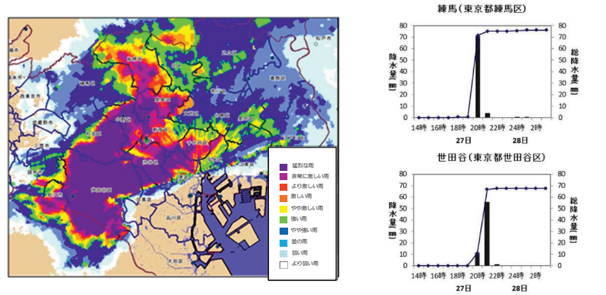
図表 2-13 2018（平成30）年8月27日の東京アメッシュ画像（左）、 気象庁雨量計データ（右） 出典：東京管区気象台「平成30年8月27日の大雨に関する東京都気象速報」
