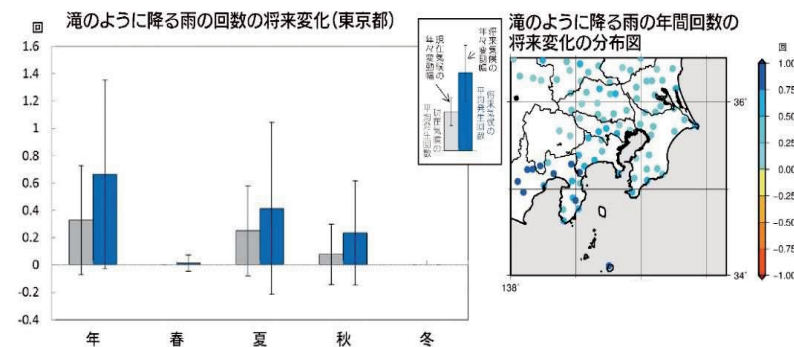
図表 2-17 気温上昇が最大の場合における1時間50ミリ以上の降雨回数の変化
