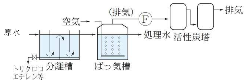
図 2-20 ばっ気法
