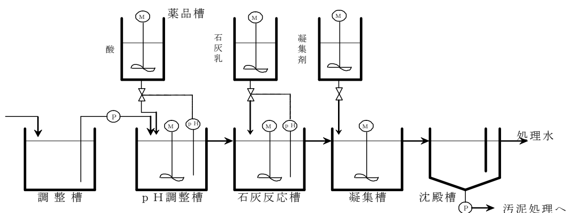
図 2-12 ピロりん酸銅の処理
