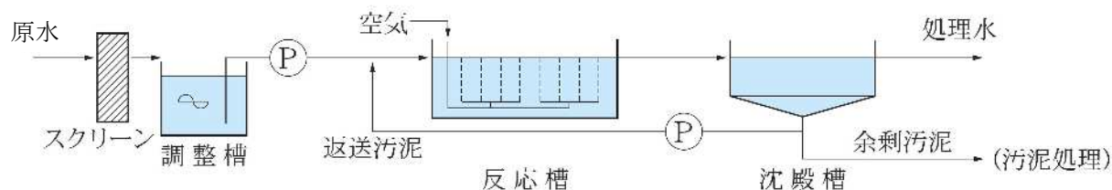
図2-6 活性汚泥法
