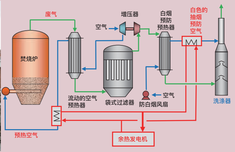
▲余热发电流程
