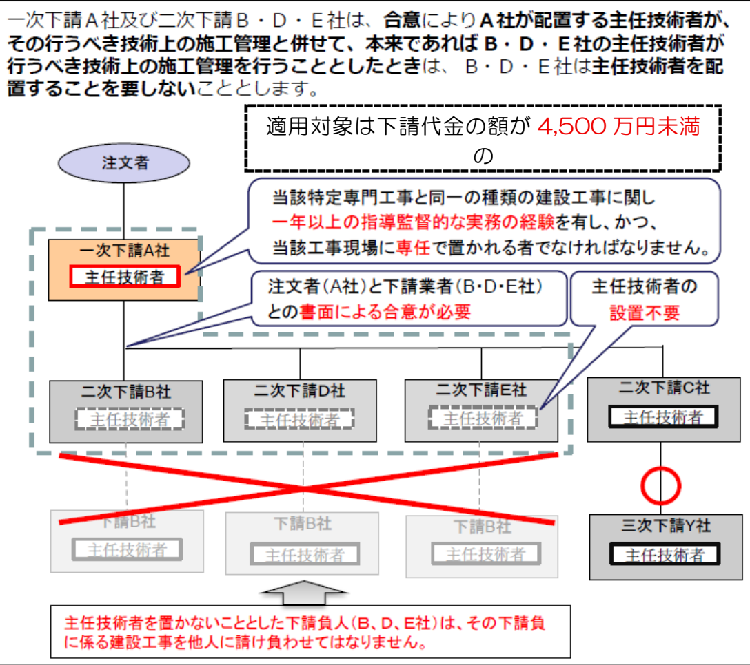
図 5 - 3 : 特定専門工事を適用した場合
