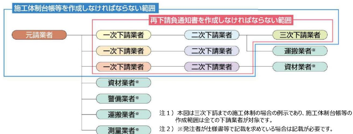
図5-1：施工体制台帳の作成すべき範囲（三次下請までである場合の例） 出典：「建設業法に基づく適正な施工体制と配置技術者」国土交通省 近畿地方整備局
