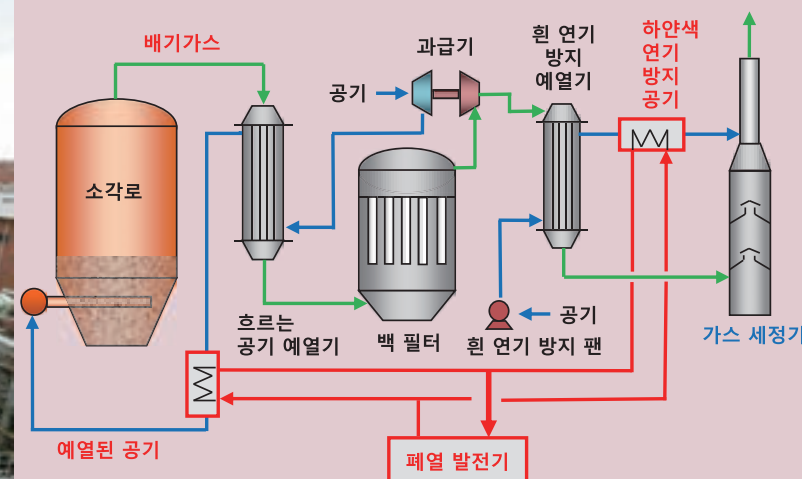
▲ 폐열을 활용한 발전 흐름
