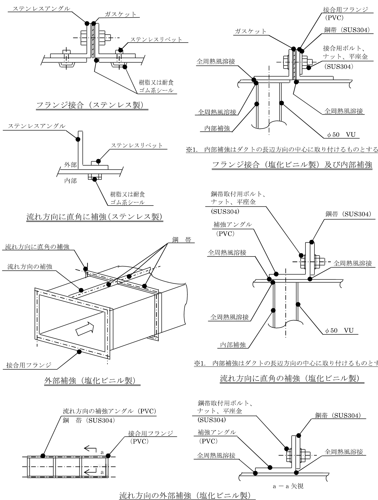
図 2.3-1 ダクト施工図 (参考図)
