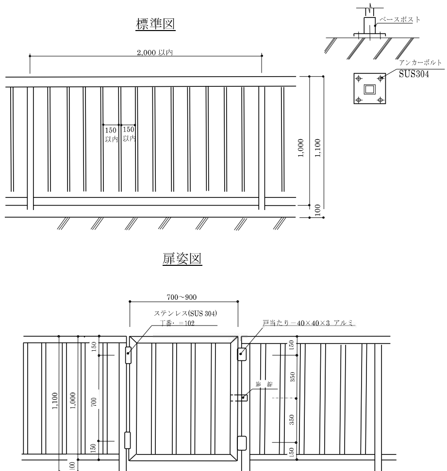
図 2.1-3 アルミ製手すりの形状
