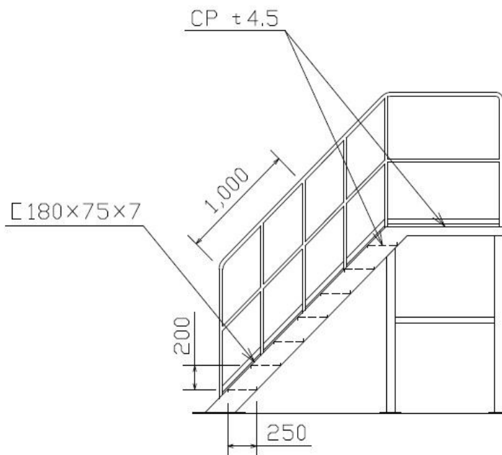
図 2.1-4 階段の形状
