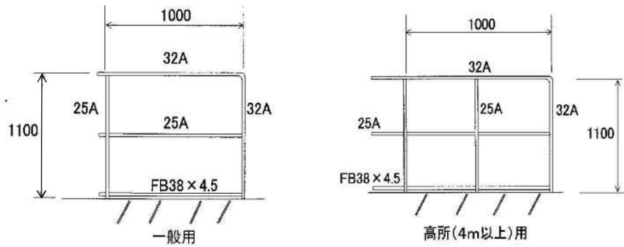
図 2.1-2 鋼製手すりの形状
