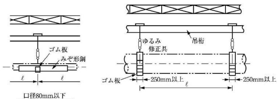
側面図 (鋼管)
