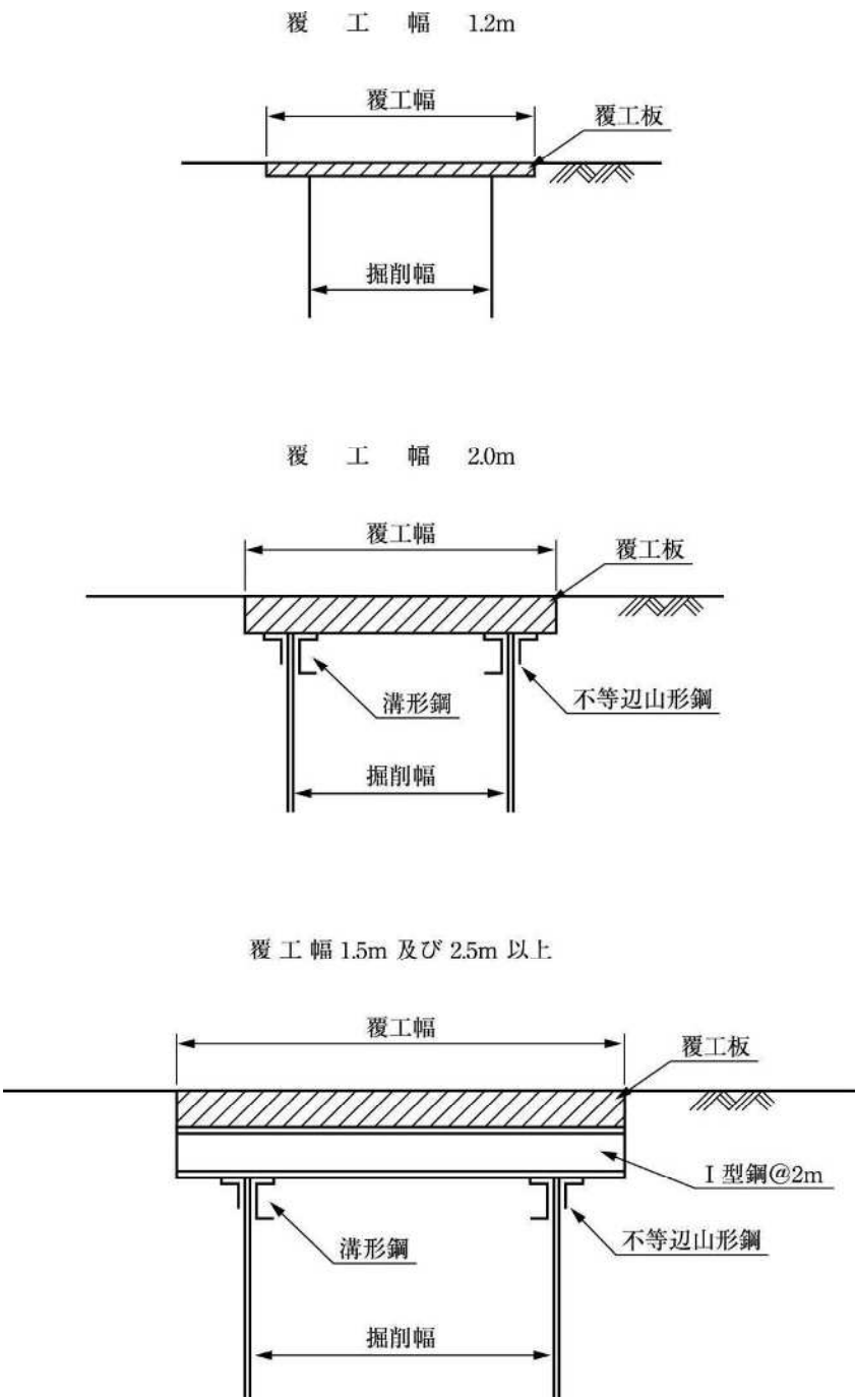
付図－6 路面覆工標準仮設図
