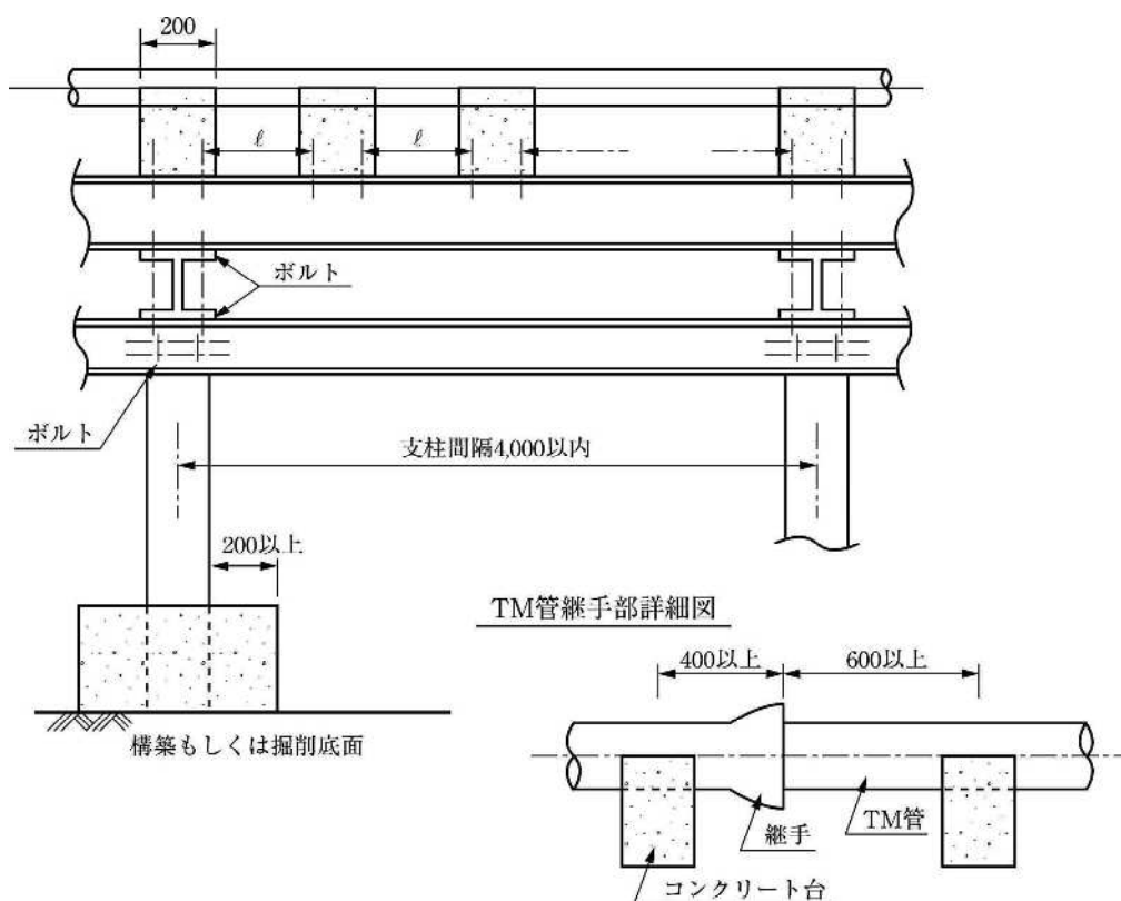
支柱間隔 4 m 以内の場合
