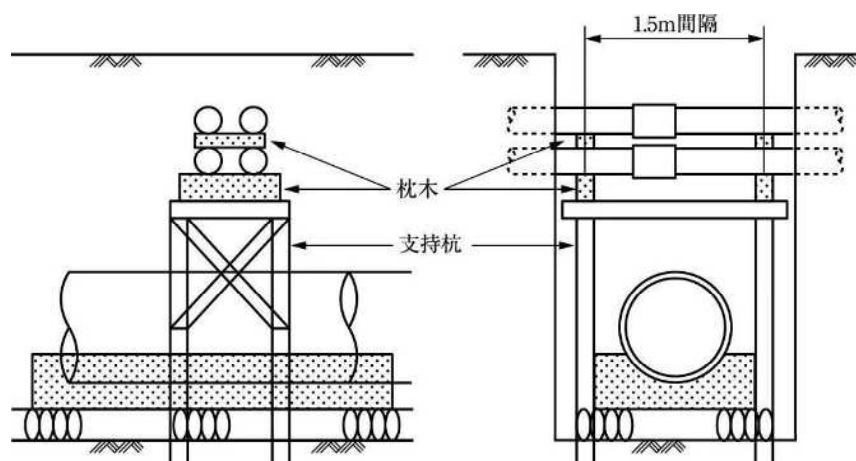
参図－２ 受け防護の設置例
