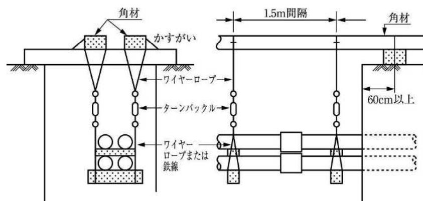
参図－１ 吊り防護の設置例
