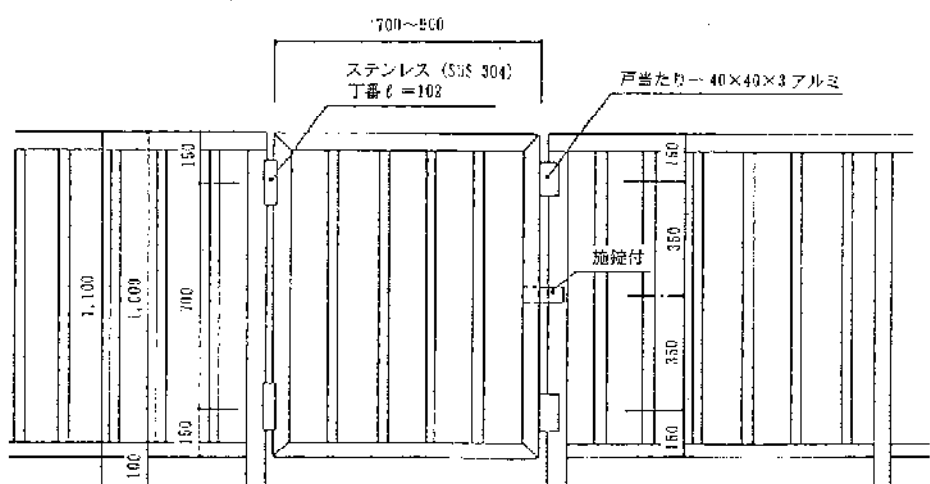
扉姿図
