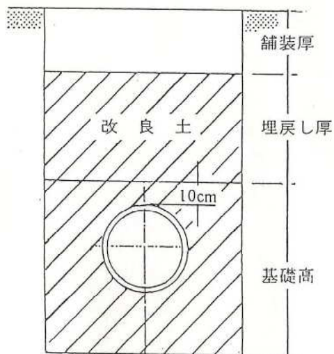
360° 砂基礎 〔改良土〕
