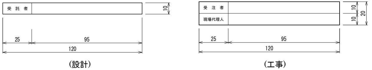
図 1-5-(2) 表題欄-2 (単位 mm)
