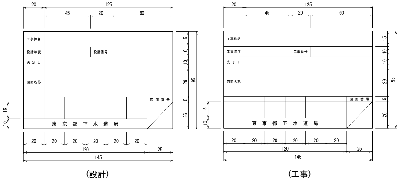
図 1-5-(1) 表題欄-1 (単位 mm)
