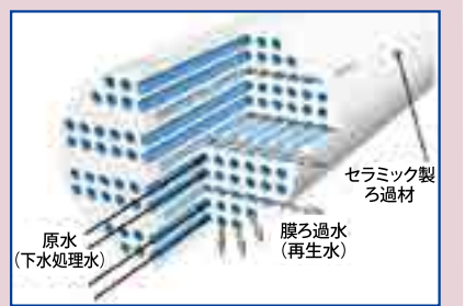
セラミック膜ろ過の構造
